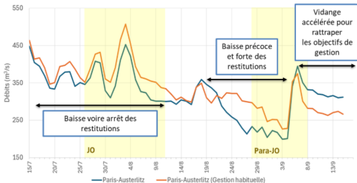
Figure 3 : Effet de la gestion des lacs sur l'abaissement du débit à Paris. Les débits mesurés à Paris-Austerlitz sont en bleu, et les débits estimés sans la gestion spécifique JO en orange montrant bien la baisse de débits opérés pendant les période JO indiquées en bandes jaune.
